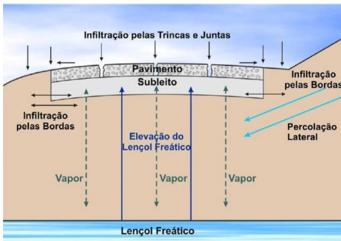
Figura 1 - Origem das águas nos pavimentos
