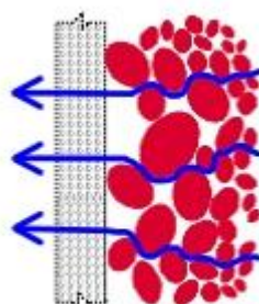
Figura 2 - Solo retido pelo geotêxtil
