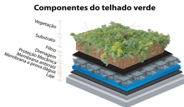
Figura 1 -Esquema de montagem para telhados verdes.
