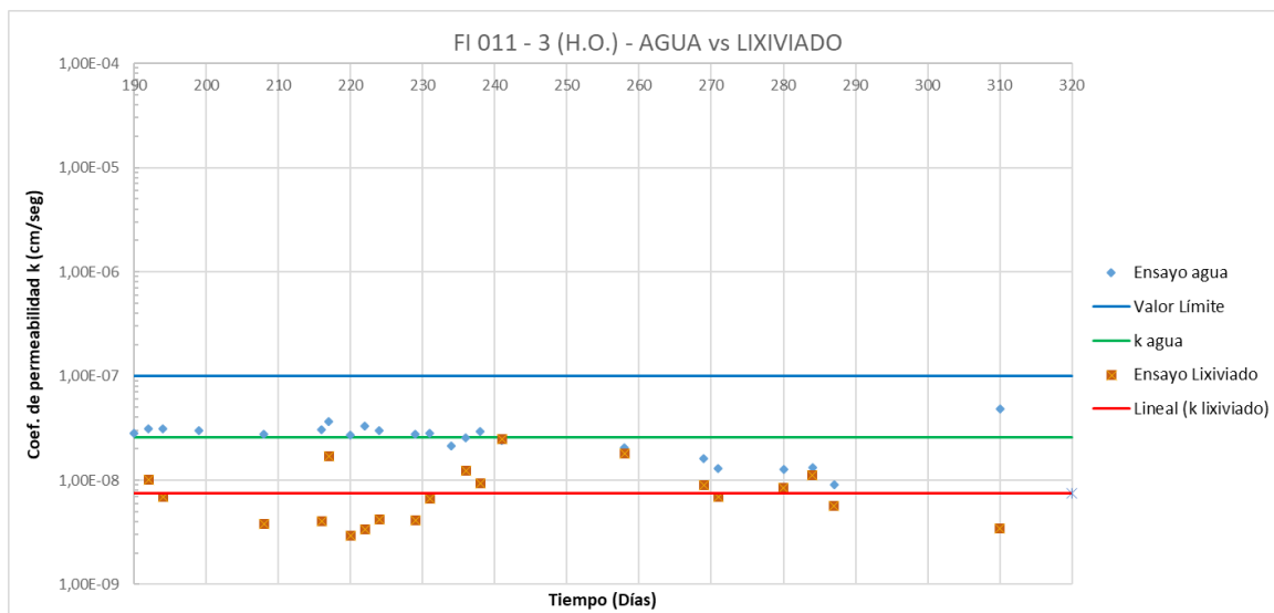
Gráfico N°2: “Comportamento Hidráulico: Agua vs Lixiviado FI-011, Próctor tipo 3, Humedad óptima”
