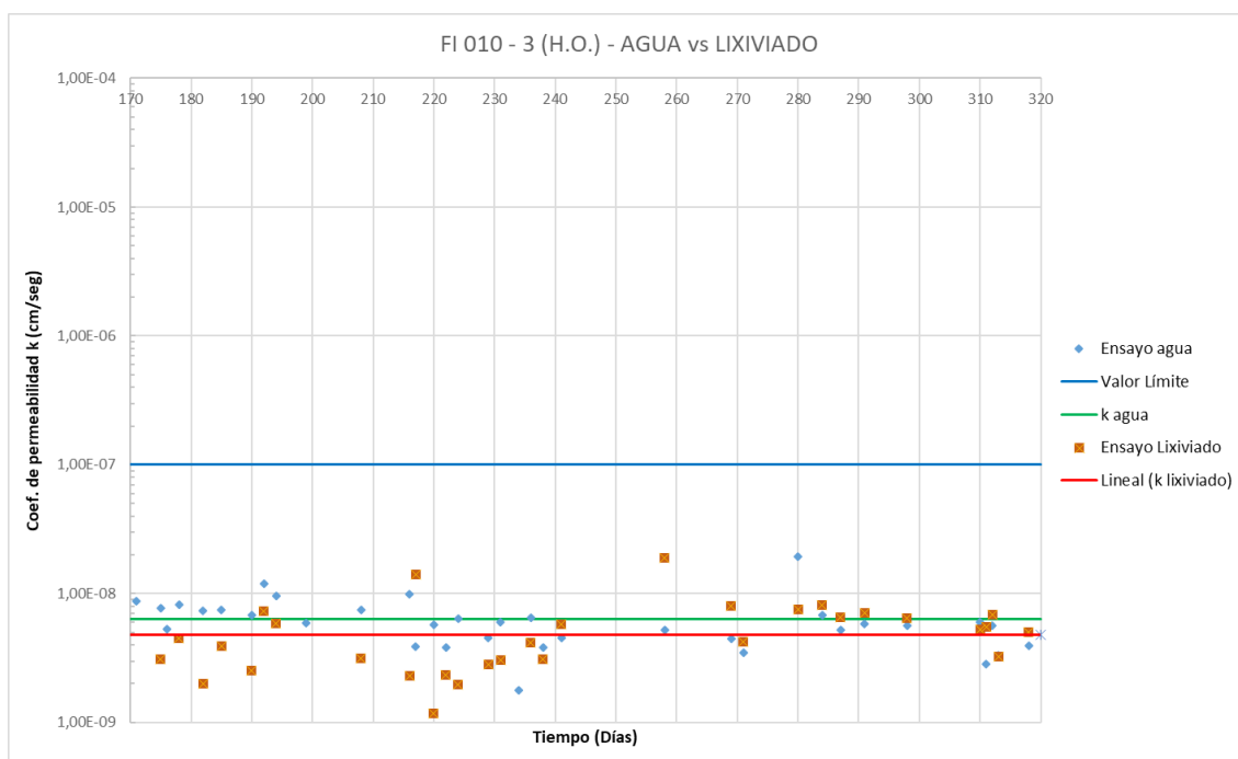
Gráfico N°1: "Comportamiento Hidráulico: Agua vs Lixiviado FI-010, Próctor tipo 3, Humedad óptima"
