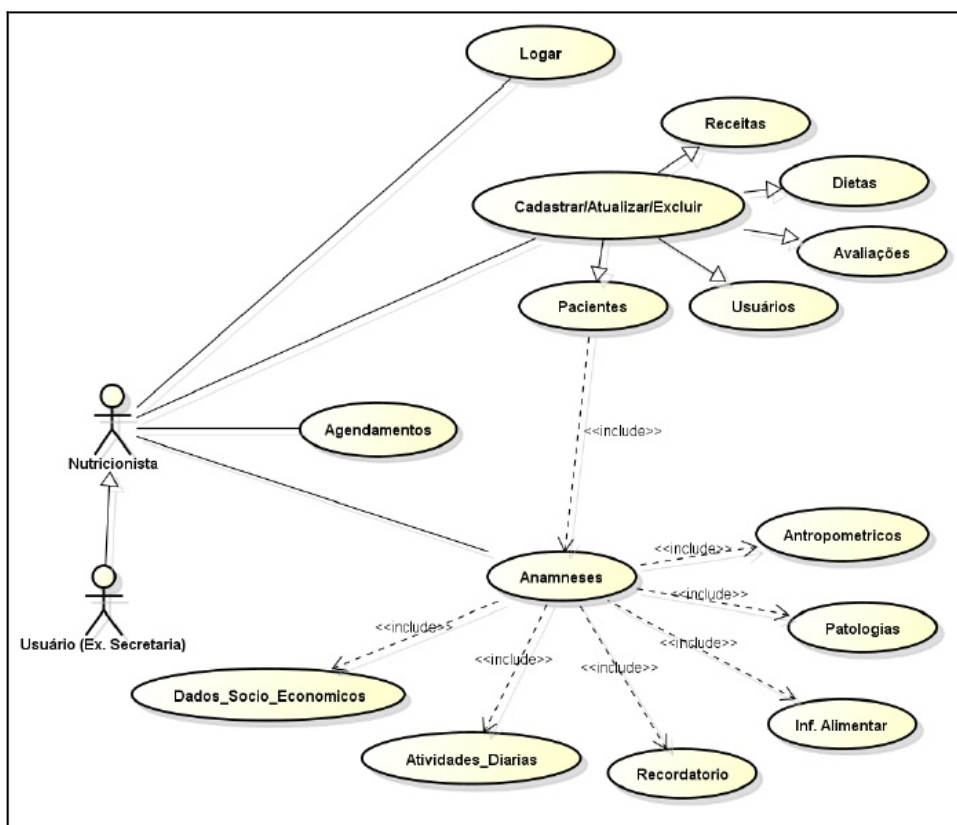
Figura 1: Diagrama Caso de uso da aplicação.
