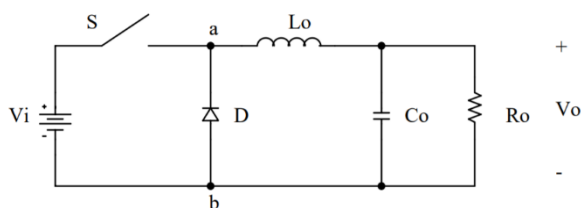
Figura 2. Topologia Buck.
